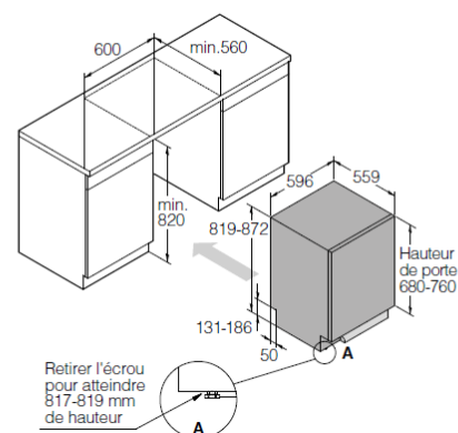
Dimensions d'encastrement
